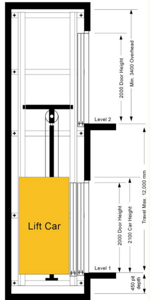
Hoistway Elevation
